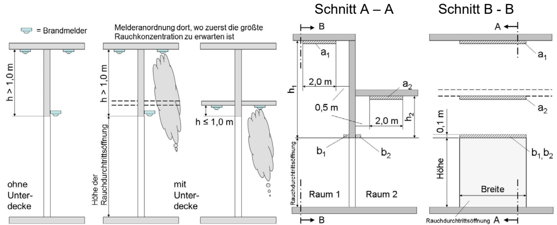
Bild 1: Maßgebende Höhe der Deckenunterfläche Bild 2: Installationsbereiche
