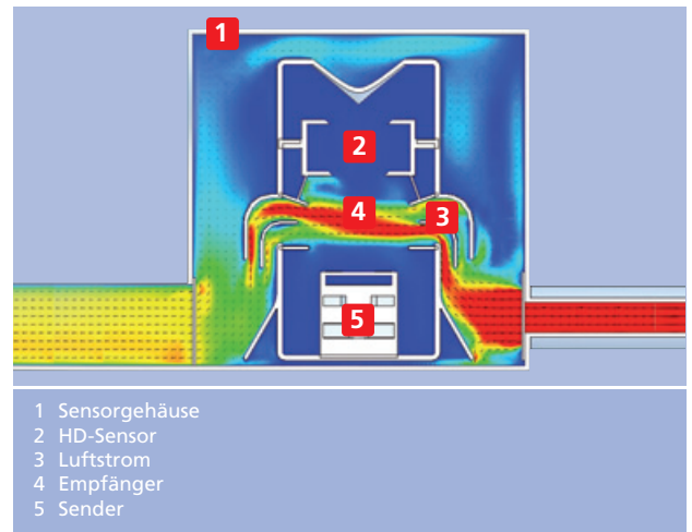
Querschnitt eines HD-Sensors im ASD 535
