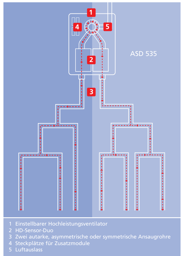
Schematischer Aufbau
